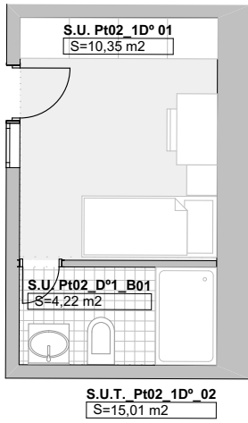
PROTOTIPO 1P 1:100
