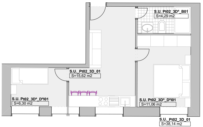
PROTOTIPO 3P°
