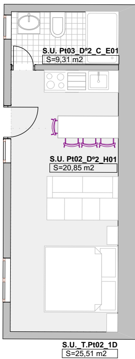
PROTOTIPO 2P 1:100
