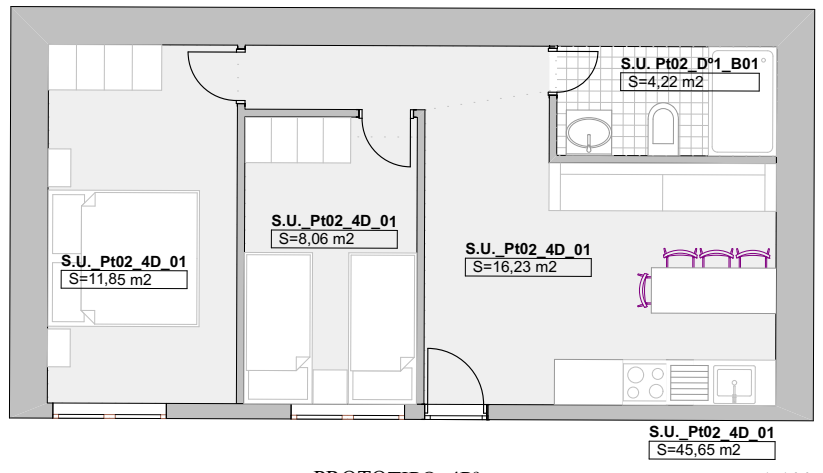
PROTOTIPO 4P°
